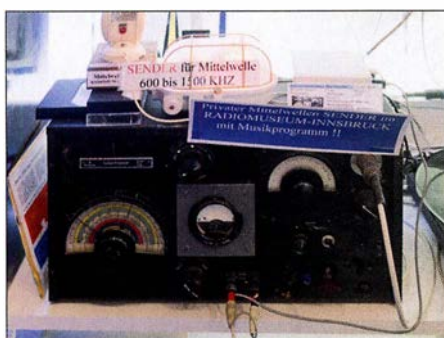
Mittelwellensender des Radiomuseums Schuchter
