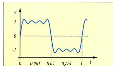
Bild 3: Nahezu rechteckförmiges Signal im Zeitbereich
