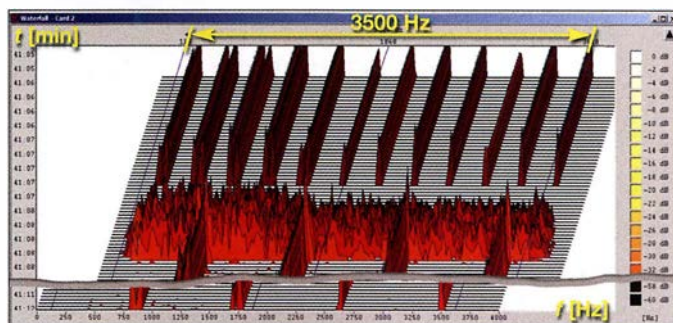
Bild 2: Chinesisches Breitbandradar auf 21 MHz im Spektrogramm
