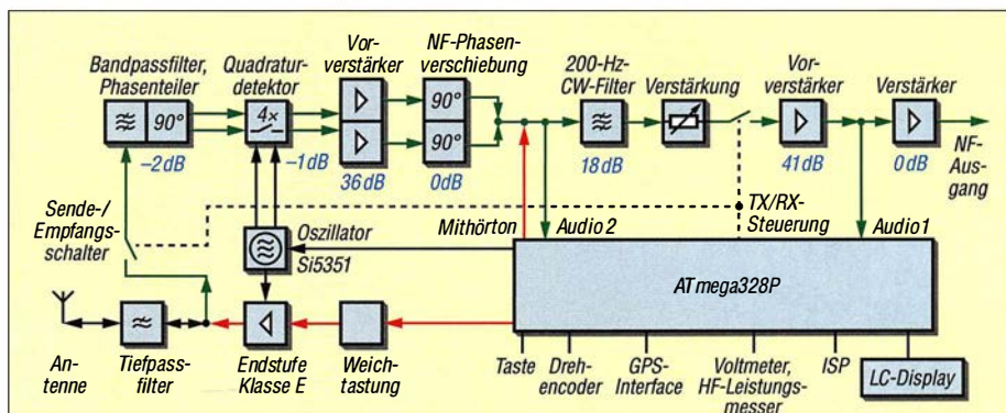
Bild 2: Blockschaltbild des Transceivers QCX; Sendezweig rot, Empfangszweig grün, gemeinsam genutzt schwarz
