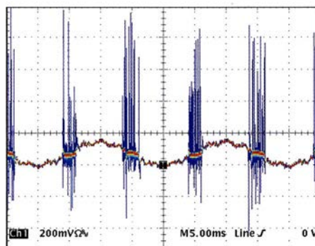
Bild 19: Das Ansmann-Schaltnetzteil liefert immer dann, wenn die Netzgleichrichterdioden leitend sind, typische Störpakete mit U_{SS} = 1,2 V im Abstand von 10 ms.
