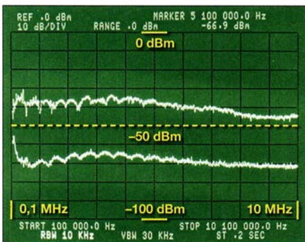
Bild 18: Störspetren der Schaltnetzteile von Ansmann (oben) und Friwo (unten) im Frequenzbereich von 100 kHz bis 10 MHz
