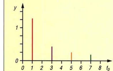
Bild 5: Frequenzspektrum des rechteckförmigen Signals in Bild 4
