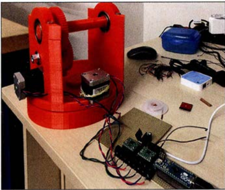
Bild 3: Testaufbau des Portabelrotors mit Schrittmotoren und angeschlossener Steuerelektronik
