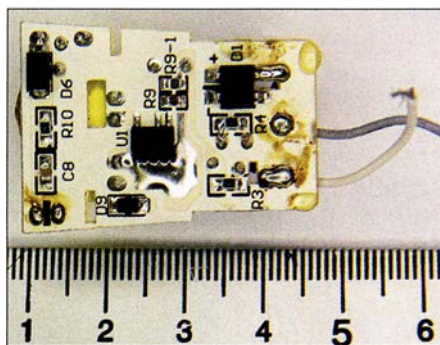
Bild 29: ... und in der Ansicht von unten
