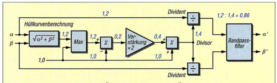
Bild 16: Basisband-Clipper mit Überkompensation der Überschwinger; die Reste der Überschwinger sind so klein, dass sie nicht mehr stören. Die ALC der Endstufe spricht nicht mehr an, die Endstufe kann die volle Leistung abgeben. Die Zahlen sollen beispielhaft die Funktionsweise des Basisband-Clippers als Überschwingersteuerung verdeutlichen.
