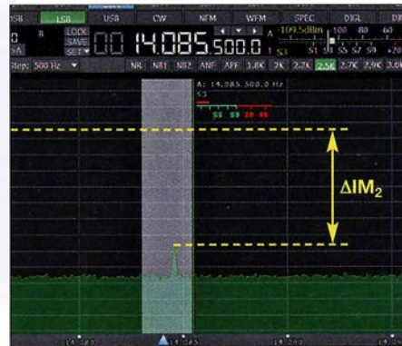
Bild 10: ... erzeugen ein IM_2 -Produkt im 20-m-Band.
