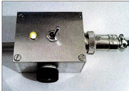
Bild 5: Fertig aufgebaute Abstimmhilfe während des Betriebs; gut zu erkennen sind der PTT-Schalter und der Einstellknopf für die Sendeleistung.
