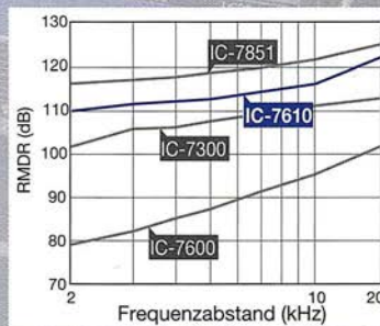
Erstauhnliche 110 dB* RMDR * repräsentativer Wert bei 2 kHz Frequenzabstand, CW und 500 Hz Bandbreite
