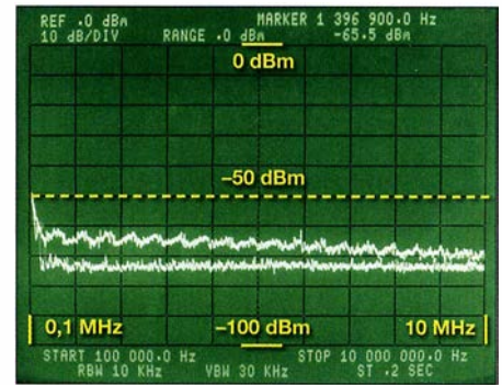
Bild 26: ... der dimmbaren LED-Lampe Philips B38
