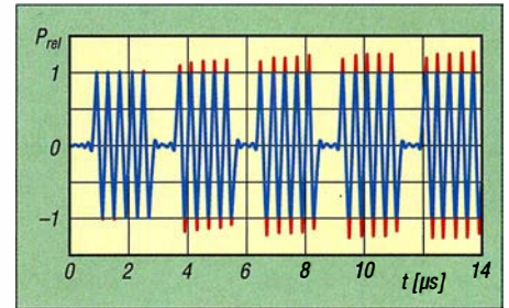
Bild 6: Einfluss der Höhe des Beschneidens beim Clipping auf die Grundschwingung bei 0 dB, 3 dB, 6 dB, 10 dB und „unendlich“
