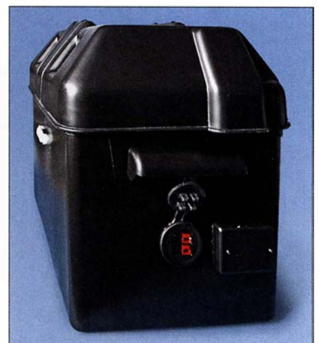
Bild 3: Stabile Kunststoffbox für die Akkumulatoren mit Anderson-Powerpole-Anschlüssen und Sicherungskästchen
