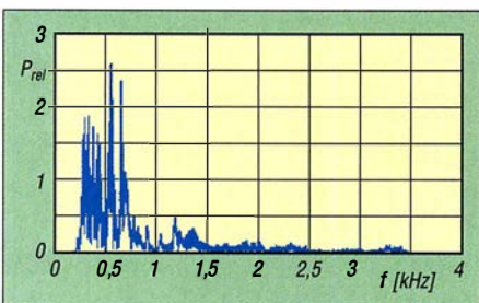
Bild 3: ... und dessen Leistungsspektrum im Frequenzbereich
