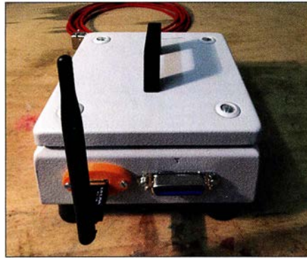
Bild 4: Die abgesetzte Steuerbox des Antennenrotors hat ein Stahlblechgehäuse, das Störstrahlungen wirkungsvoll dämpft.
