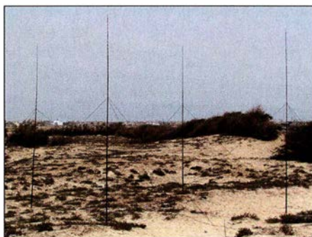
Das 4-Square für 40 m bestand aus vier 12 m hohen Spiderbeam-Glasfasermasten.
