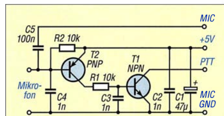
Bild 7: Zusatzschaltung für den direkten Anschluss des Lautsprechermikrofons an den Yaesu FT-817
