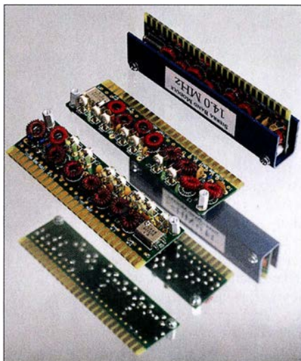
Bild 4: Markenzeichen des Sierra sind die Steckmodule für die einzelnen Amateurbänder. Sie enthalten Ein- und Ausgangsfilter sowie einen Quarz.
