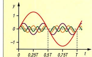
Bild 4: Signalbestandteile des rechteckförmigen Signals in Bild 3
