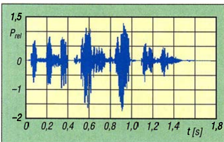
Bild 2: Gewöhnliches Sprachsignal im Zeitbereich ...
