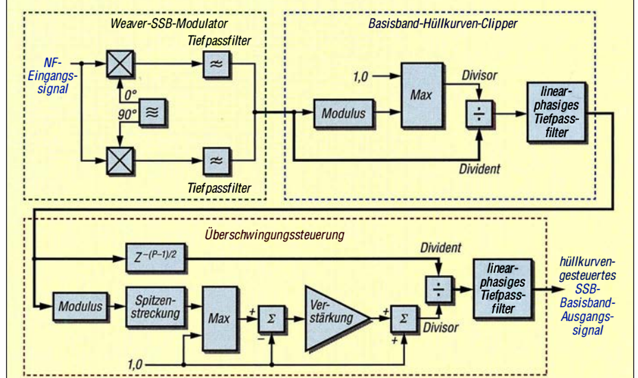
Bild 17: Komplettes CESSB-System; die dicken Linien bedeuten eine parallele Bearbeitung in zwei Kanälen.
