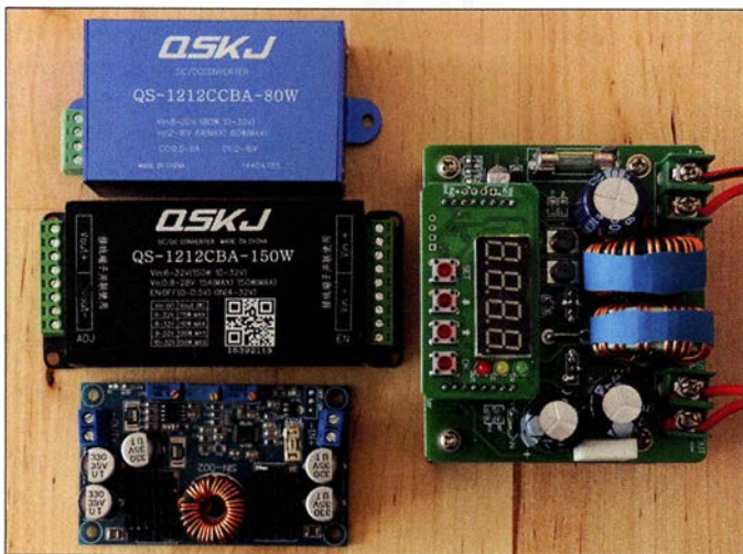
Bild 6: Einige der von uns getesteten Gleichspannungswandler; letztlich eingesetzt wurde der QS-1212 CCBA-80W, der oben links zu sehen und z. B. bei Ebay erhältlich ist.
